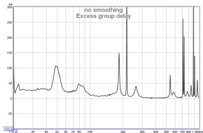
Figura 6 – Ritardo di gruppo differenziale
