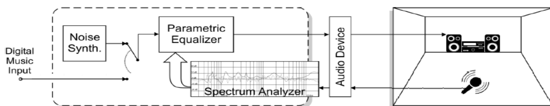
Figura 4 – Analisi della risposta al rumore
